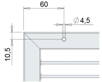
FORATURA EBA
