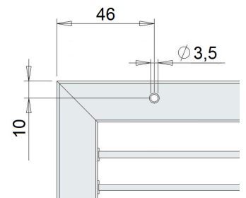
FORATURA EBV
